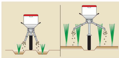
AN-60 散布イメージ
