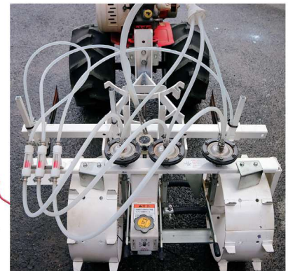
みのる土壌消毒機は10L、20Lの丸缶・角缶に対応。 (FI-3・FI-21を除く)
