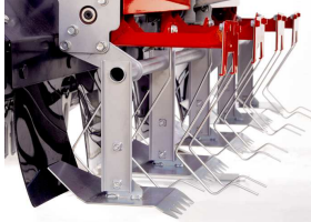
株間除草用の揺動ツース
