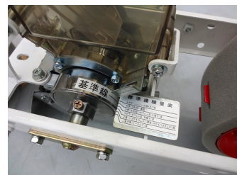
繰出ロールで播種量調節
