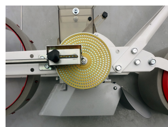
ピッチ調節板で株間調節
